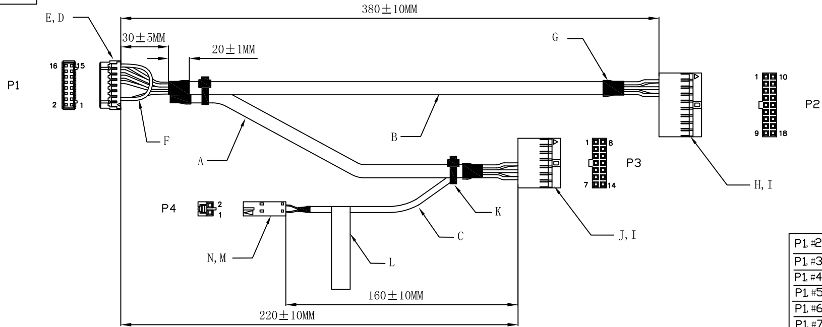
PIN WIRING
