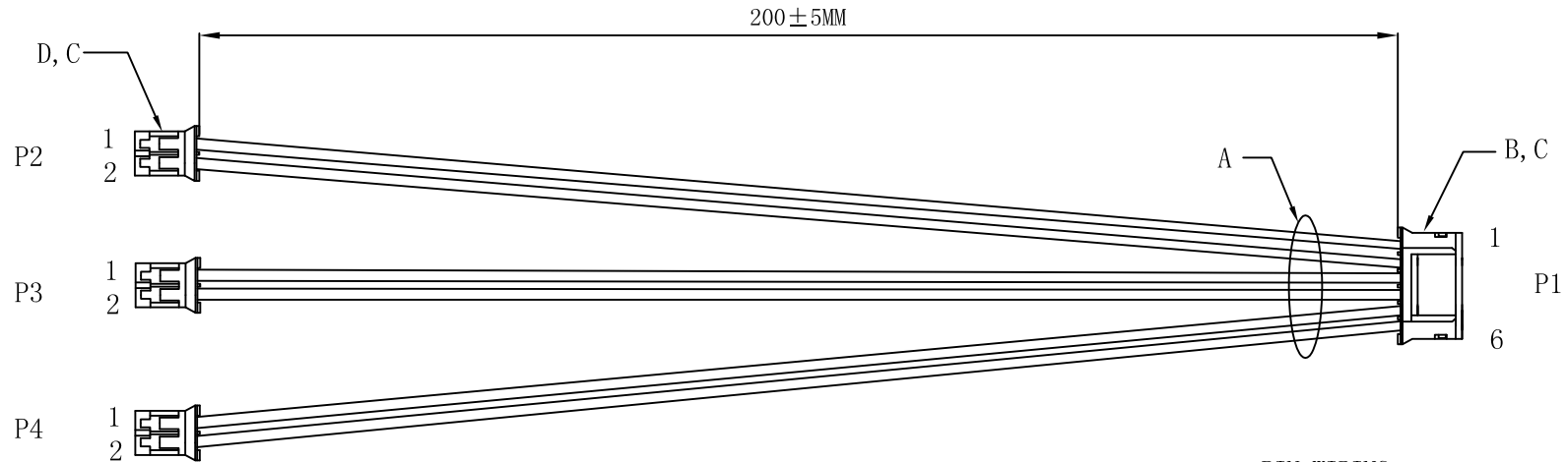
PIN WIRING
